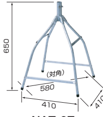
NAT-3Z
