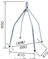
NAT-2Z
